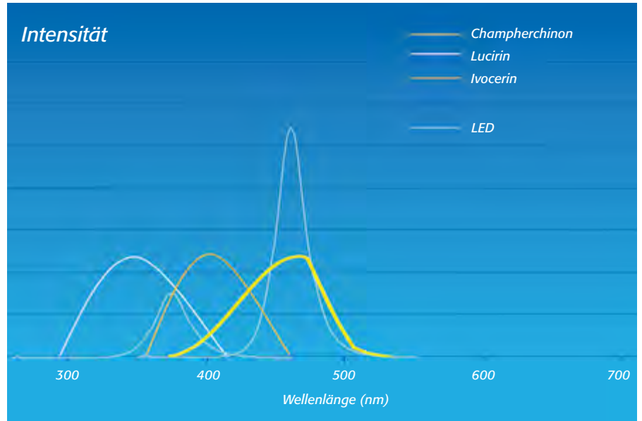
Abb. 1 Absorptionsspektren der Photoinitiatoren und Emissionsspektren der Lichtgeräte
