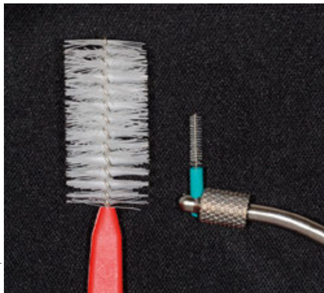
Abb. 6: Die Extreme des derzeitigen Größenspektrums. Links: IDBG-R, Top Caredent, PHD = 5,2 mm; rechts: CPS 06 prime, Curaden, PHD = 0,6 mm.
